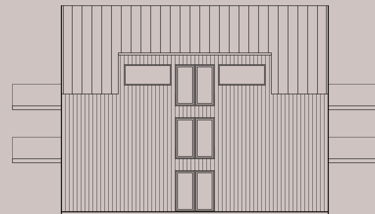
Fasad Öster
